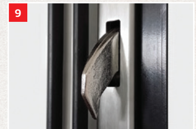
VK3 3-Punkt-Sicherheitsverriegelung mit 2 Massivschwenkriegeln
